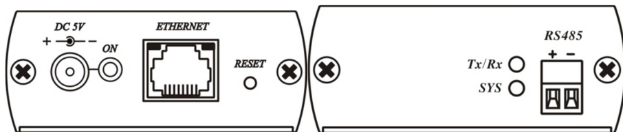
Рис.3 Разъемы и индикаторы SC1415
