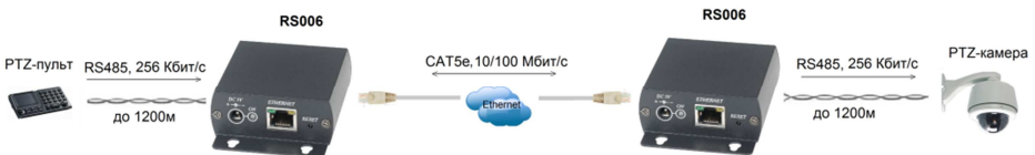
Рис. 3 Схема подключения SC1415
